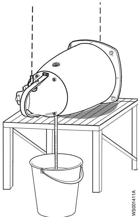
Afbeelding 22: Met koelmantel
