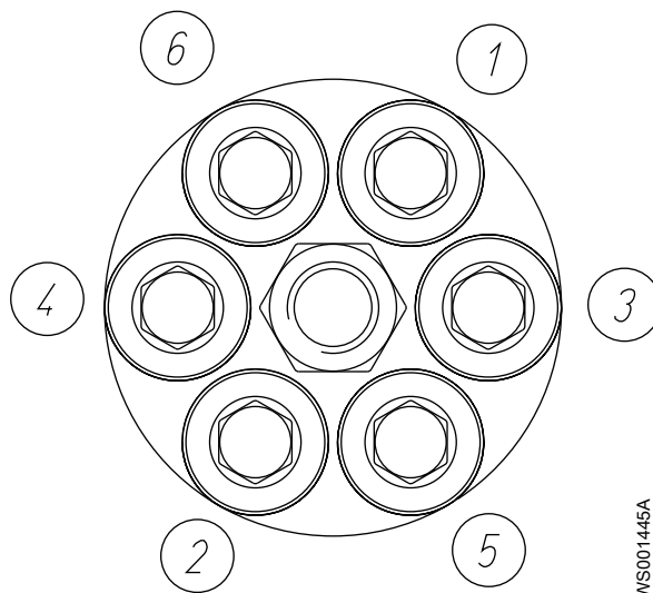
Afbeelding 26: Sterpatroon voor randschroeven
