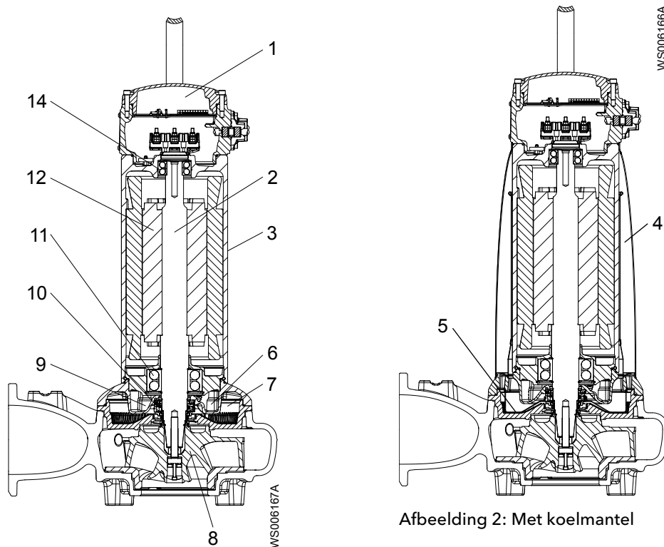
Afbeelding 1: Zonder koelmantel
