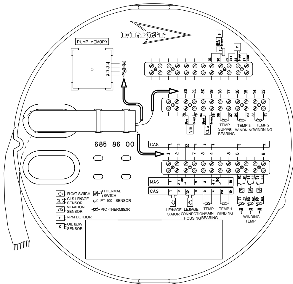
Afbeelding 12: MAS 711, de pijlen geven de nummers van de SUBCAB-kabeldraden aan.
