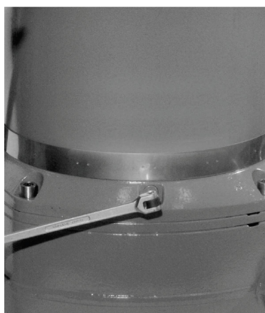
Afbeelding 18: Met koelmantel
