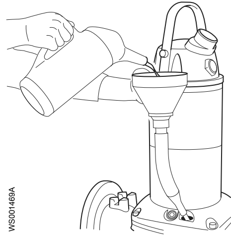
Afbeelding 25: Zonder koelmantel
