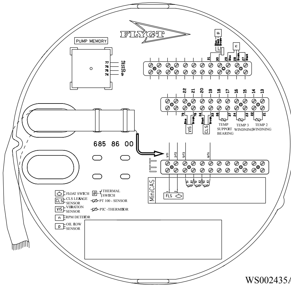
Afbeelding 14: MiniCAS en thermistors
