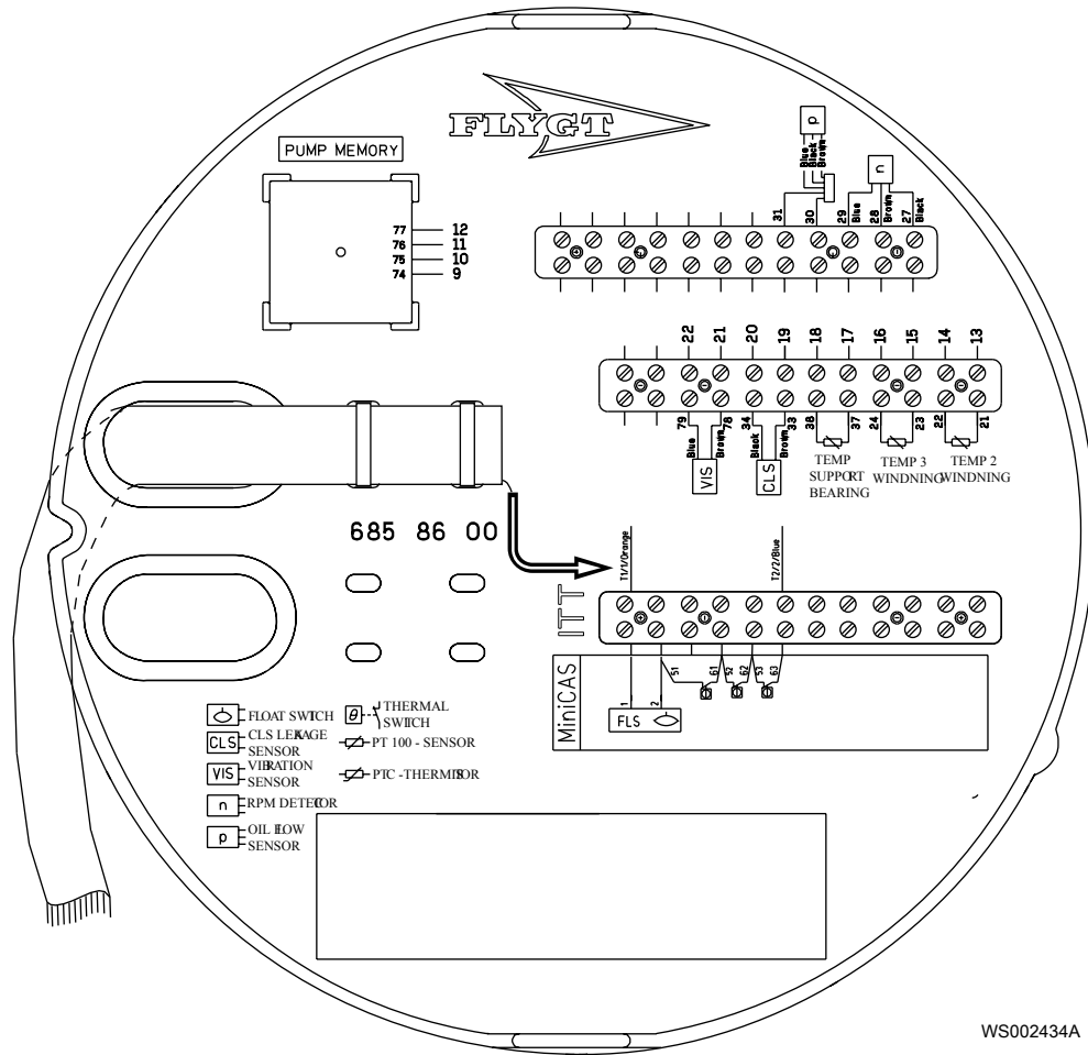
Afbeelding 13: MiniCAS en thermocontacten
