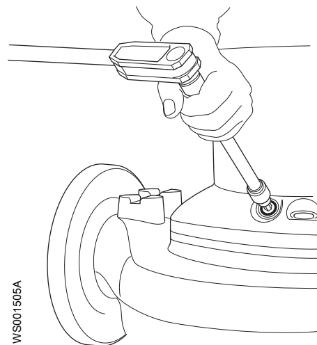
Afbeelding 19: Zonder koelmantel
