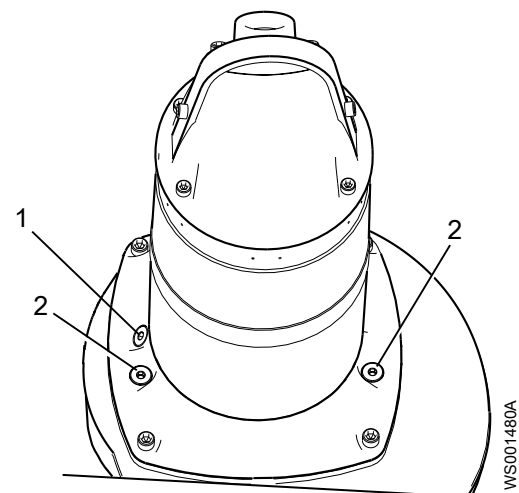
Afbeelding 17: zonder koelmantel
